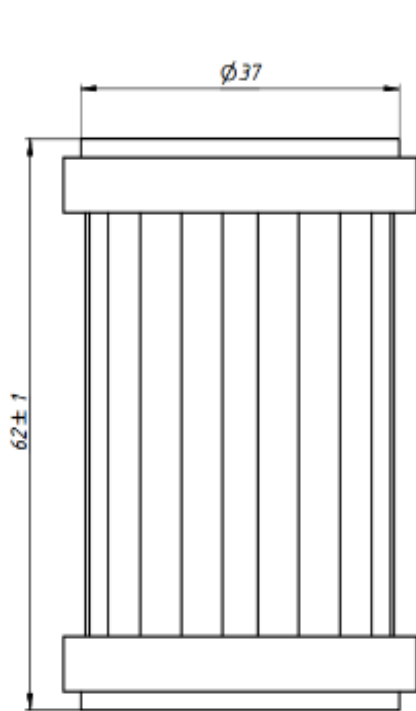
SF131-4407040 Элемент фильтрующий
